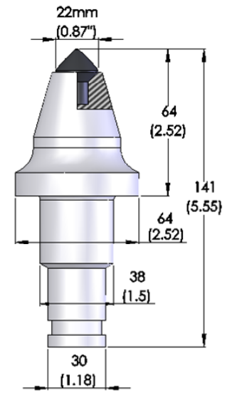
7. JZ64/38-TS41C/M22-23-3
