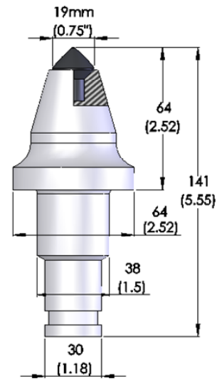
6. JZ64/38-TS40C/M19-23-3
