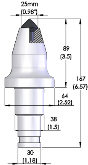
5. JZ64/38-TS5C/Z19-23-3
