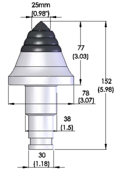
6. JZ77/38-WSMX/Z25-42N-3
