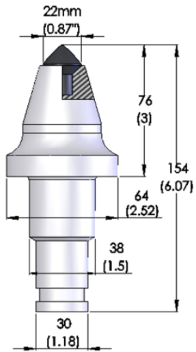
4. JZ76/38-TS32C/M22-23-3
