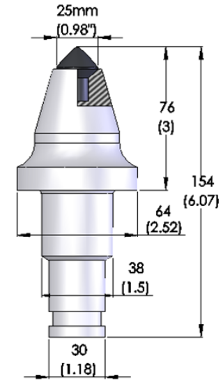
7. JZ64/38-TS41C/M22-23-3
