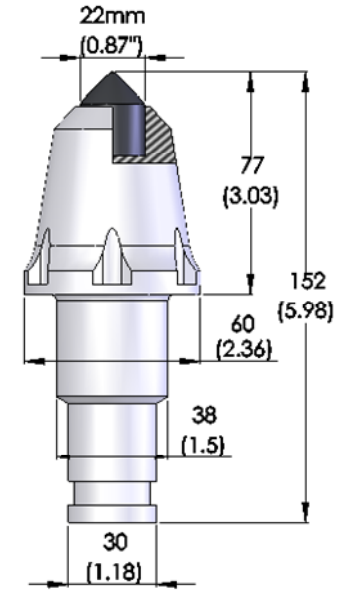
6. JZ77/38-WSMX/Z25-42N-3
