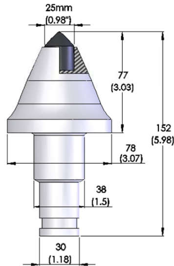
5. JZ77/38-WSMX/Z25-23-3
