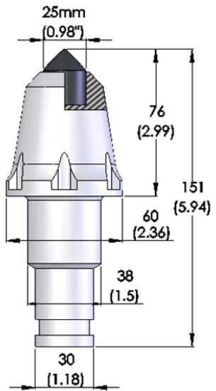
4. JZ77/38-WSM/Z25-23-3
