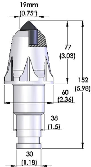
5. JZ77/38-WSMX/Z25-23-3
