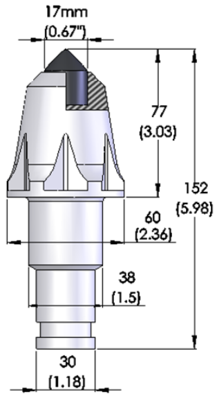
4. JZ77/38-WSM/Z25-23-3
