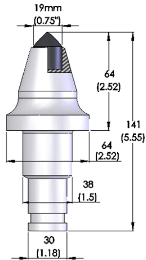
5. JZ64/38-TS5C/Z19-23-3
