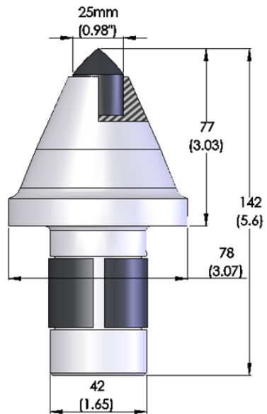
4. JZ77/42-WSM/Z25-23-3
