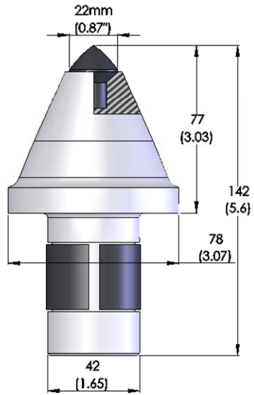
4. JZ77/42-WSM/Z25-23-3
