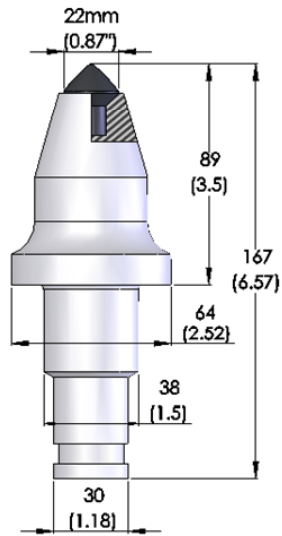
4. JZ76/38-TS32C/M22-23-3
