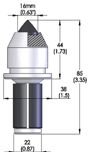
4. JZ45/20-RS17/M16-42-3
