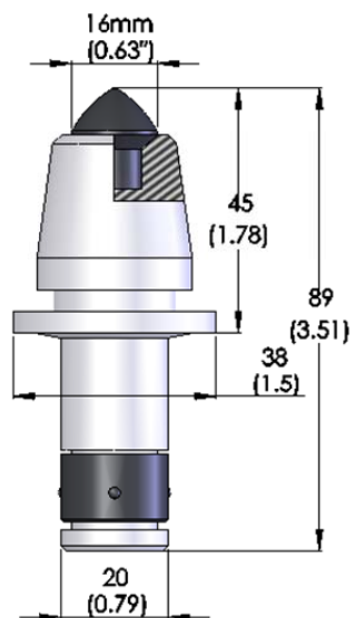
4. JZ45/20-RS17/M16-42-3
