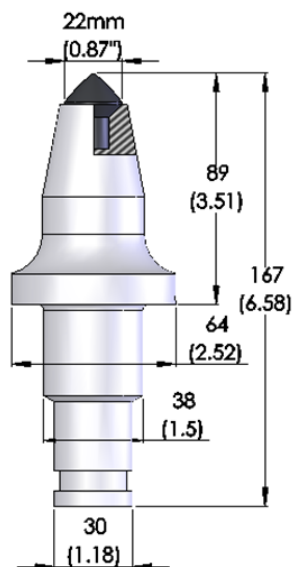
4. JZ76/38-TS32/M22-42-3
