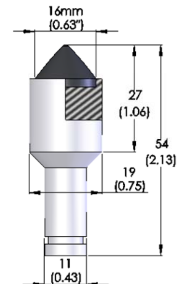
7. JZ27/11-CM42/P16-42-3
