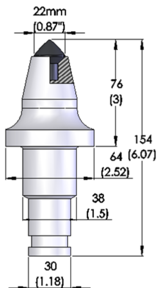
4. JZ76/38-TS32/M22-42-3
