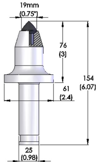
4. JZ65/25-C35R/Z16-42-3
