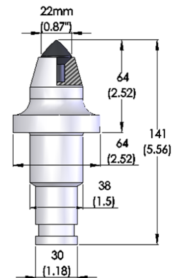
7. JZ64/38-TS41/M22-42-3
