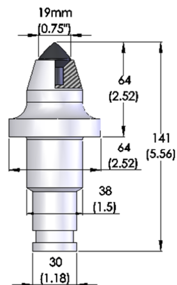
6. JZ64/38-TS40/M19-42-3
