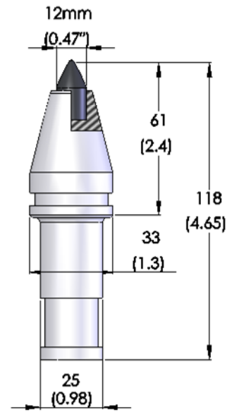
6. JZ61/25-C31HD/Z12-42-3
