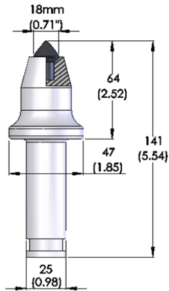
5. JZ64/25-C36R/M18-42-3
