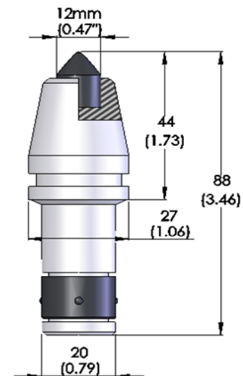
7. JZ27/11-CM42/P16-42-3
