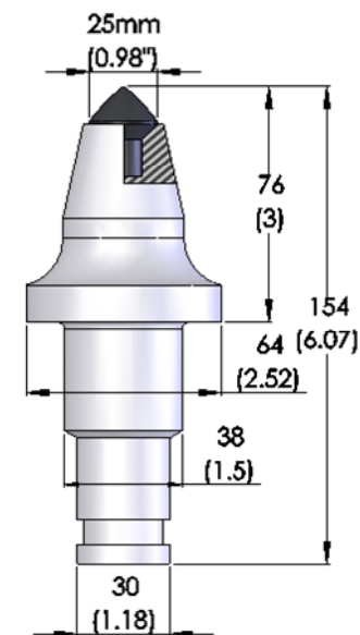
7. JZ64/38-TS41/M22-42-3
