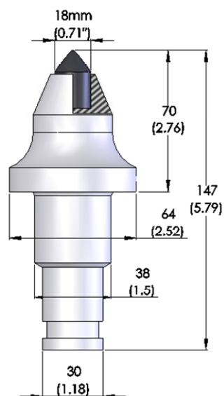
5. JZ70/38-P3DS/Z18-42-3
