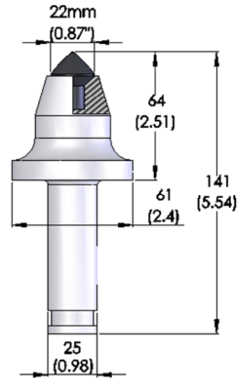
6. JZ61/25-C31HD/Z12-42-3
