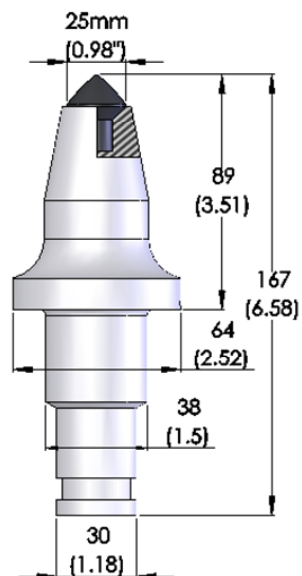
6. JZ64/38-TS40/M19-42-3
