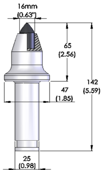
4. JZ65/25-C35R/Z16-42-3
